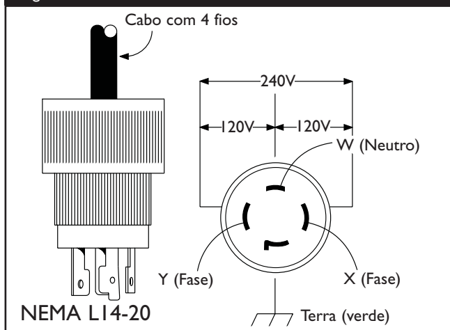
Figura 23 — Tomada com Trava 120/240 V CA, 20 A
